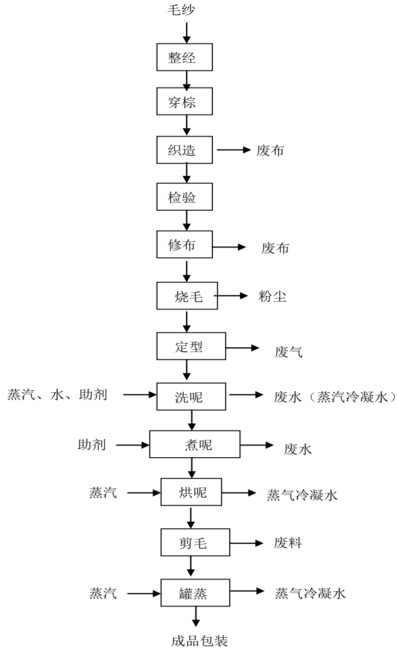
图 2.2-4 精纺面料生产工艺流程图
