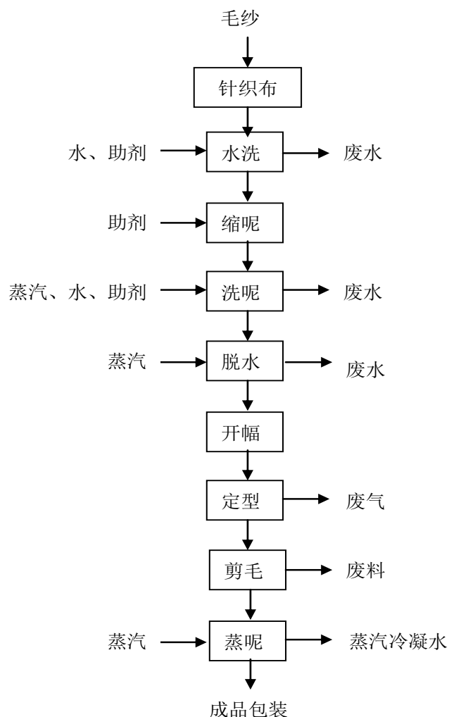
图 2.2-3 针织面料生产工艺流程图
