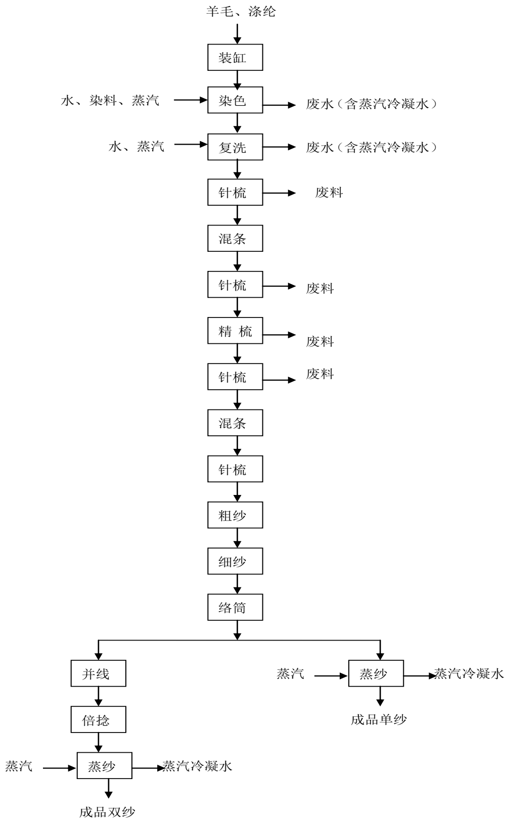
图 2.2-2 毛纱生产工艺流程图
