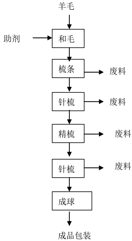
图 2.2-1 毛条生产工艺流程图
