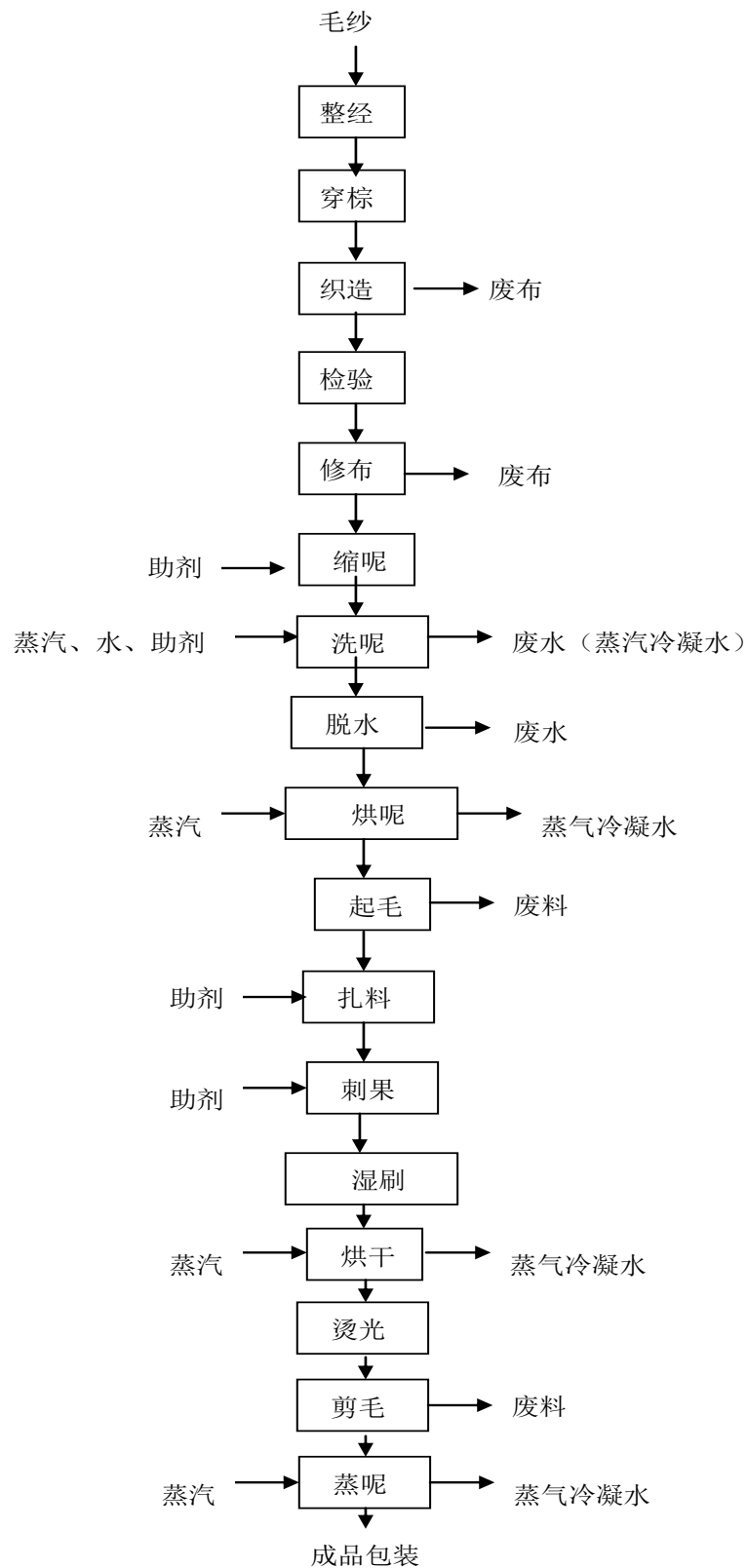
图 2.2-5 粗纺面料生产工艺流程图
